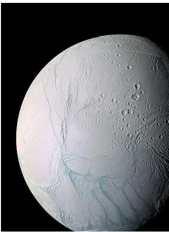
Figure 215: Enceladus
